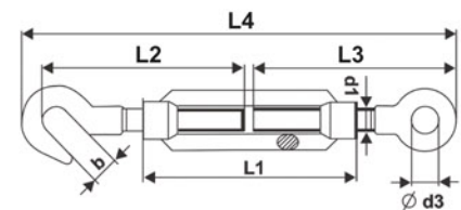
مهارکش با میل پیچ قلابدار - یک سر چشمی، یک سر قلاب (مدل A)
