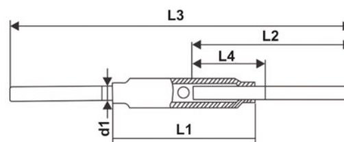
مهارکش با میل پیچ ساده
