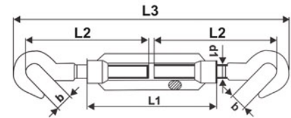
مهارکش با میل پیچ قلابدار - دوسر قلاب (مدل B)
