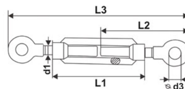
مهارکش با میل پیچ قلابدار-دوسرچشمی (مدل C)
